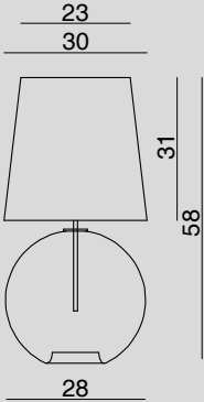
LUGIG1203 LAMPADA DA TAVOLO / TABLE LAMP Glass 1 x Ø 28 cm - Cable 200 cm 1 x E27 60 W
